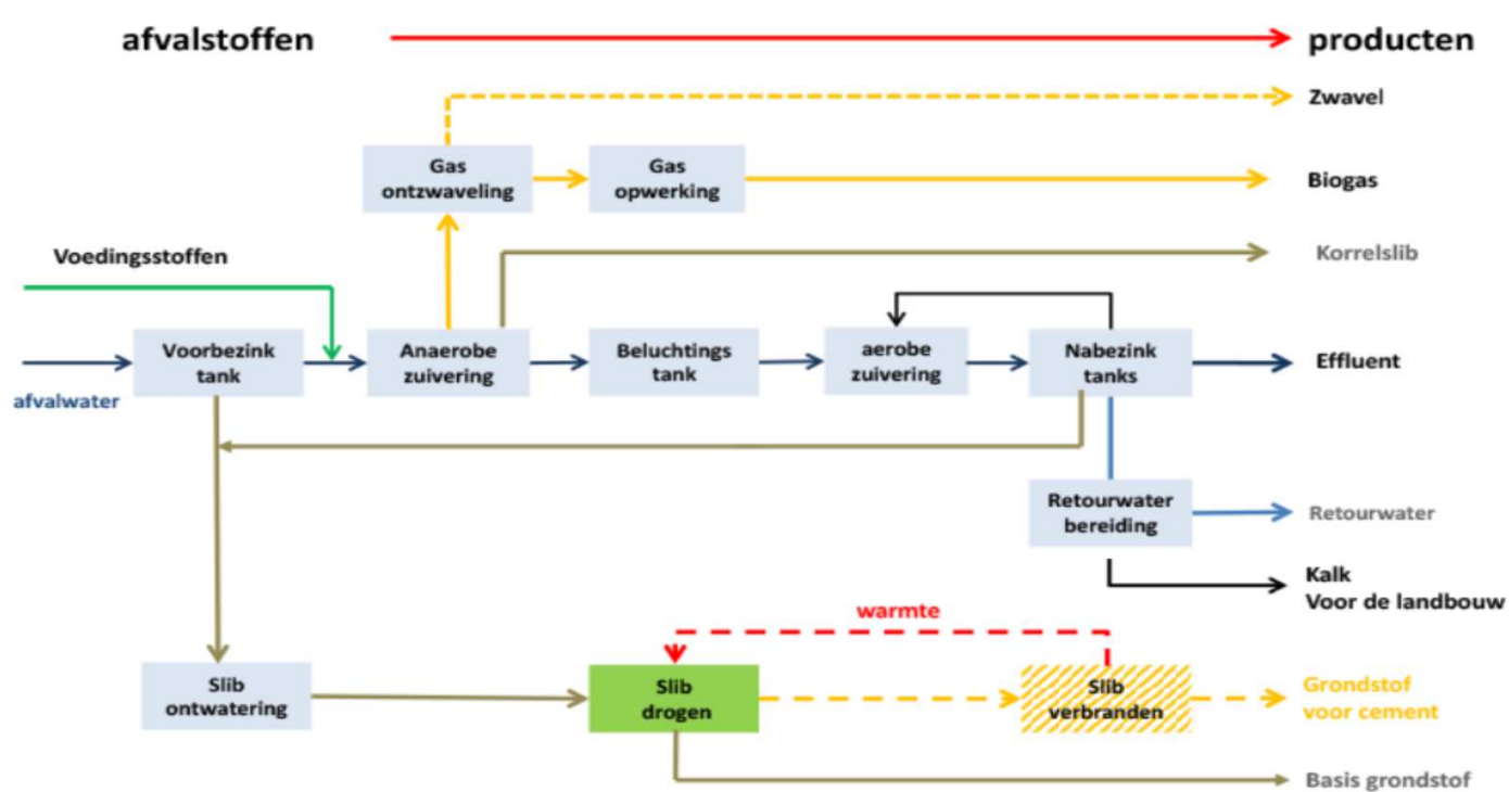
Flowschema IWE
